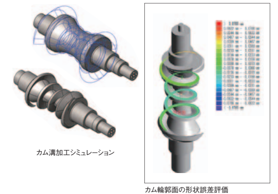
カム輪郭面の形状誤差評価
